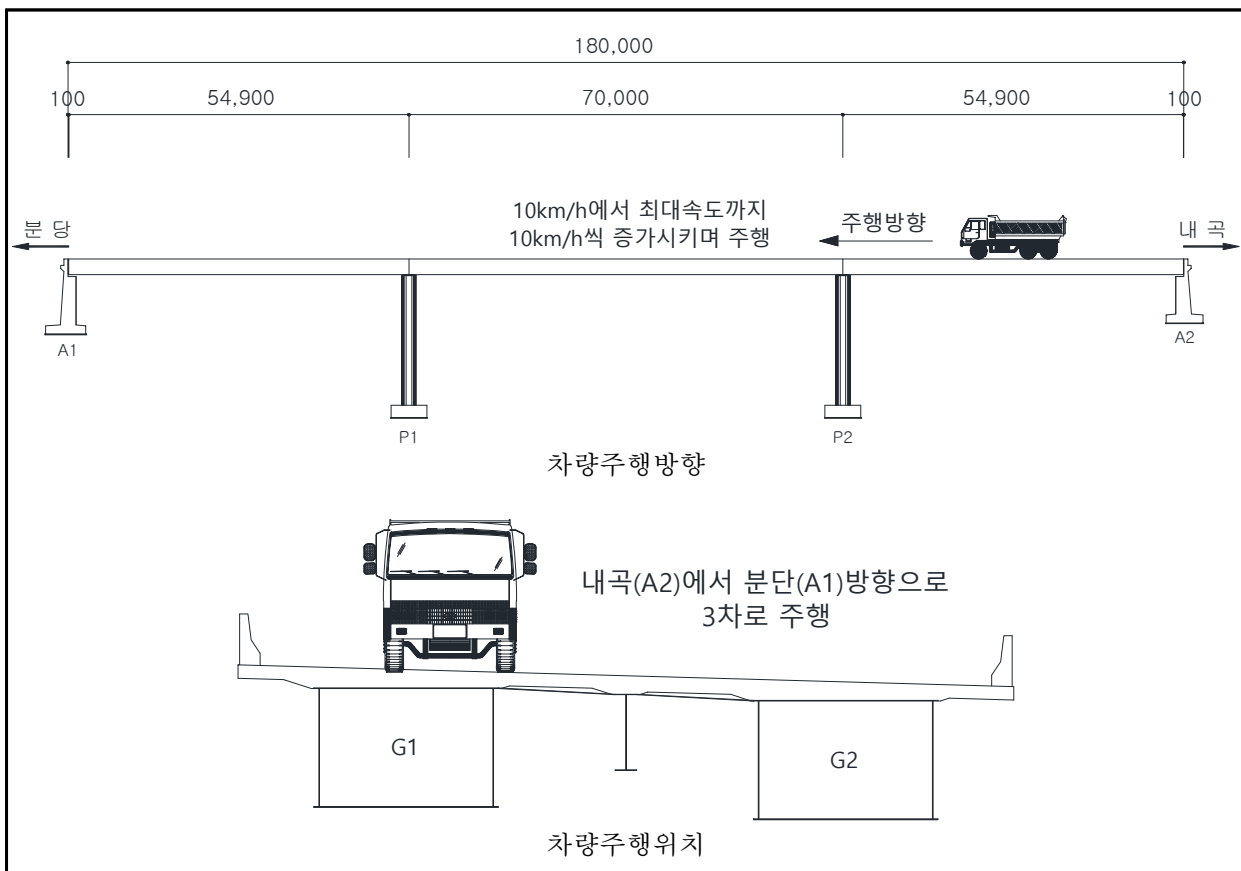
[그림 5.16] 동적주행시험 시험차량 주행위치
