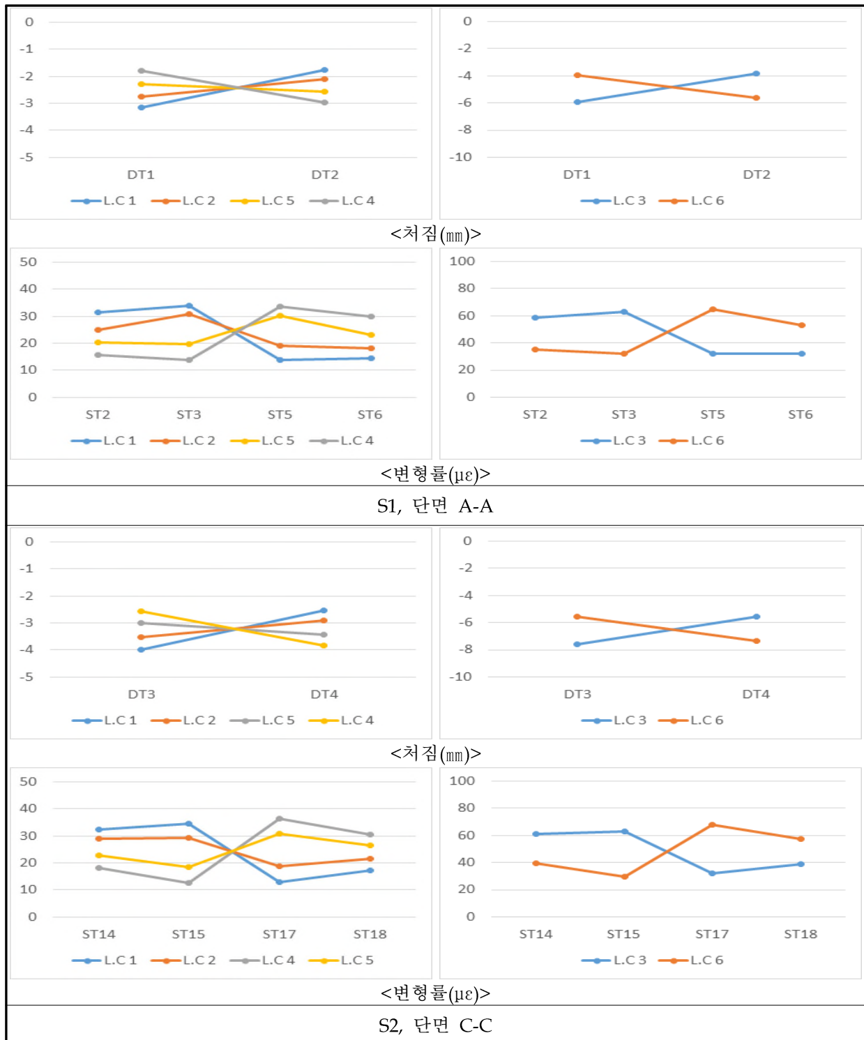
[그림 5.14] 횡방향 거동특성
