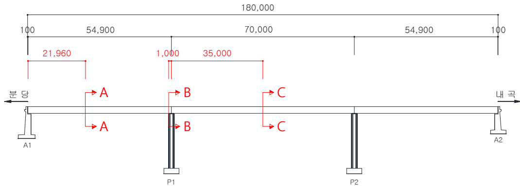
[그림 5.4] 계측기 부착 종단면 위치
