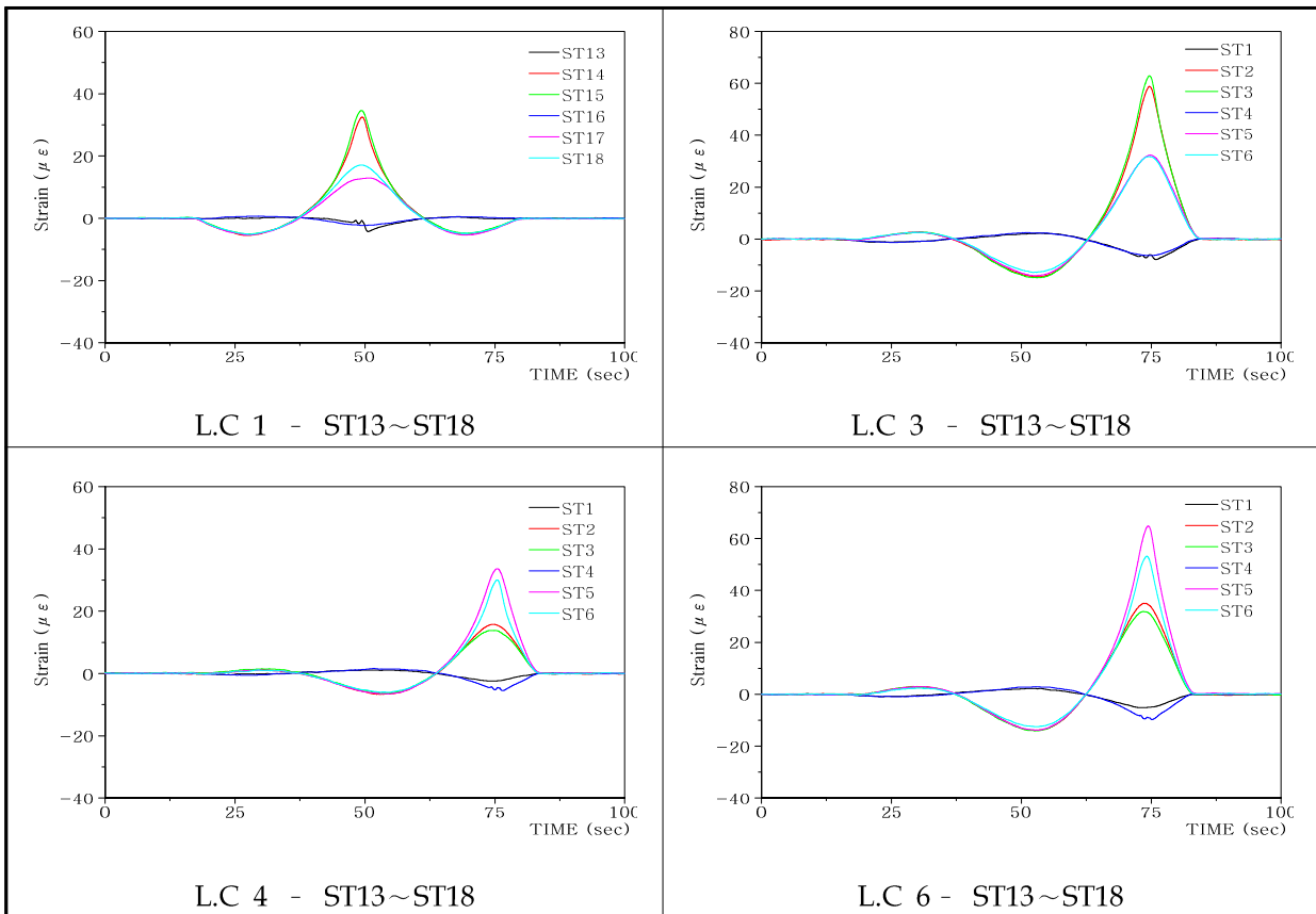
[그림 5.13] 변형률 정적 응답 Graph일레(S2, 단면 C-C)
