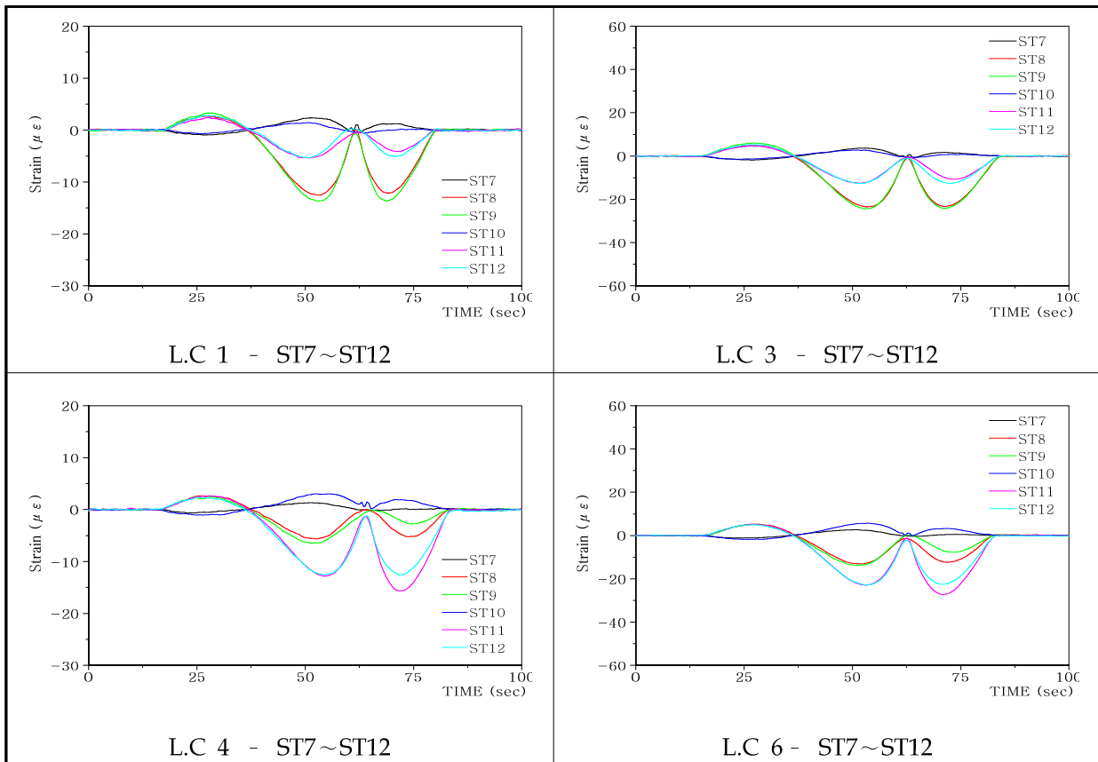
[그림 5.12] 변형률 정적 응답 Graph일례(P1, 단면 B-B)
