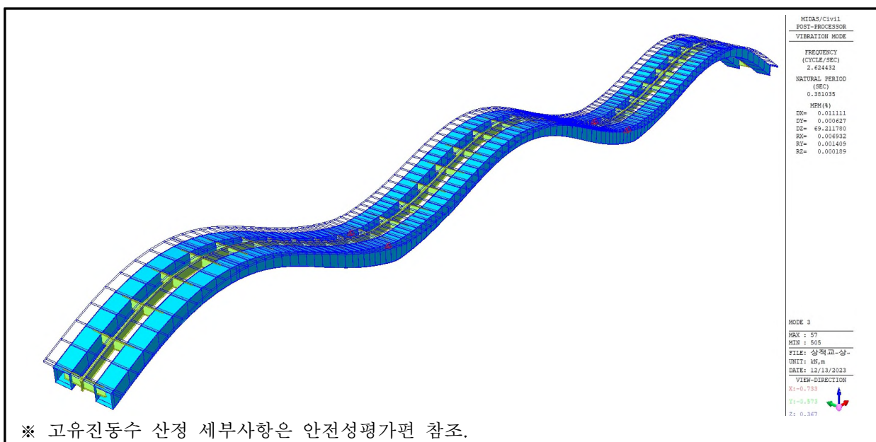
[그림 5.19] 연직 1 Mode 형상
