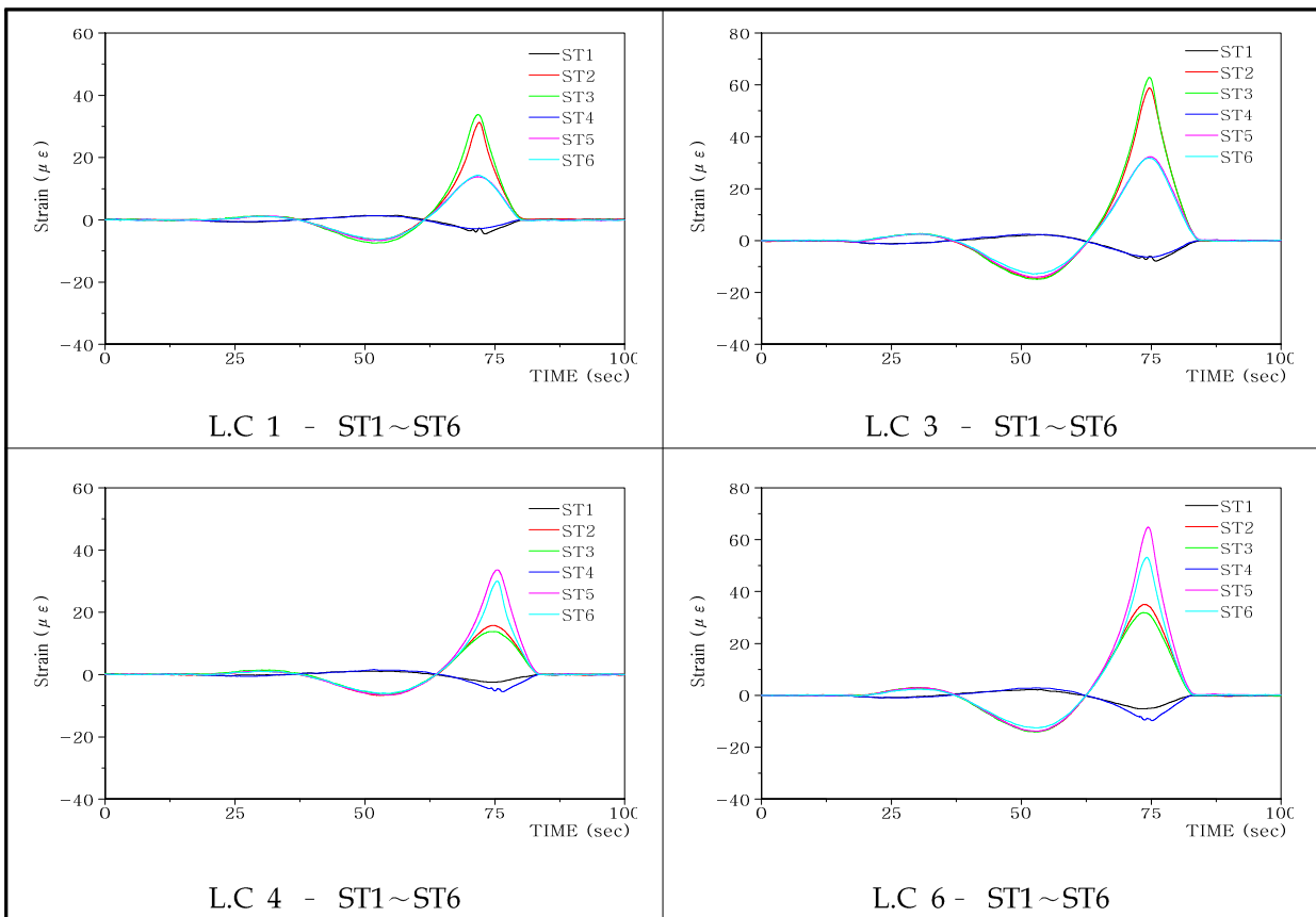
[그림 5.11] 변형률 정적 응답 Graph일레(S1, 단면 A-A)
