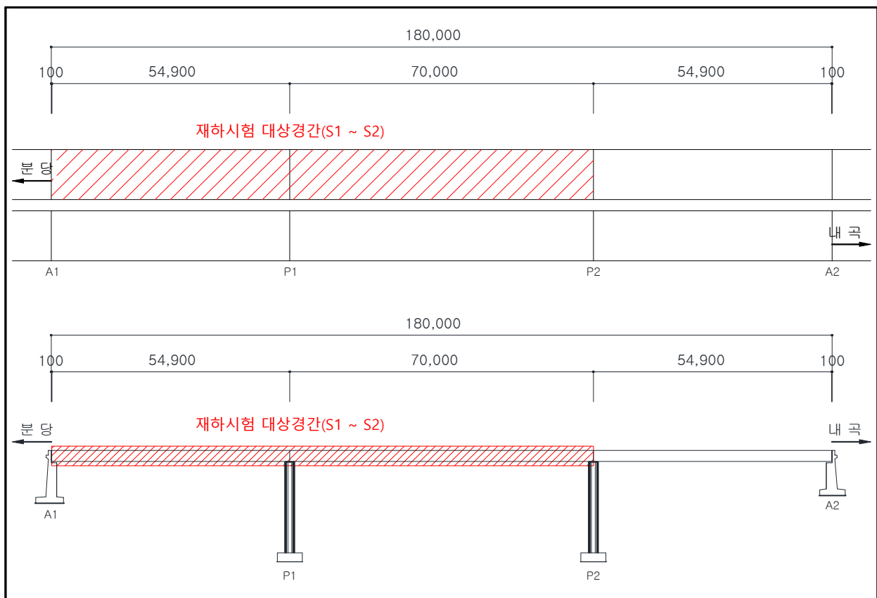
[그림 5.3] 재하시험 대상경간 및 계측기 설치 위치
